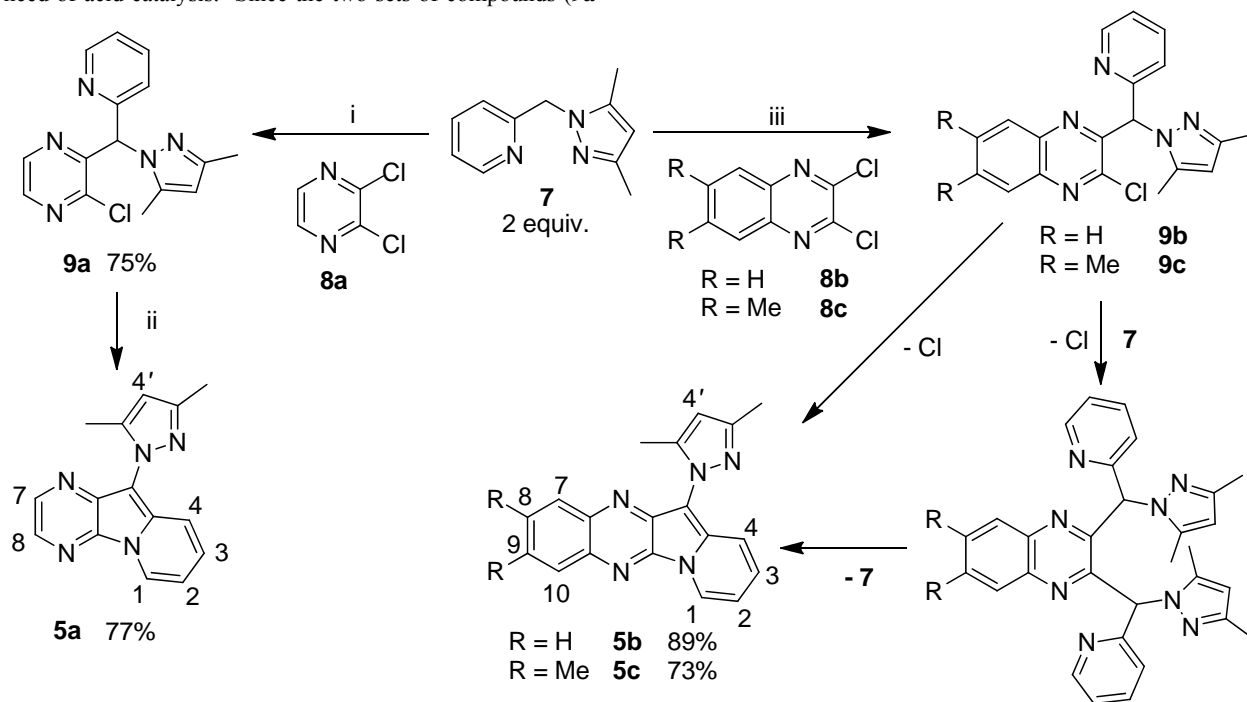
Scheme 1. i) n -BuLi, THF, -78\text{ }^{\circ}\text{C} , r.t., 9a ; ii) TFA, \text{CH}_3\text{CN} , 5a ; iii) n -BuLi, THF, -78\text{ }^{\circ}\text{C} , r.t. to reflux.
